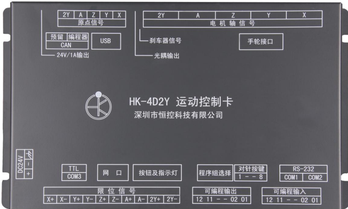
4D2Y 主板（224mm * 130mm * 42mm）
