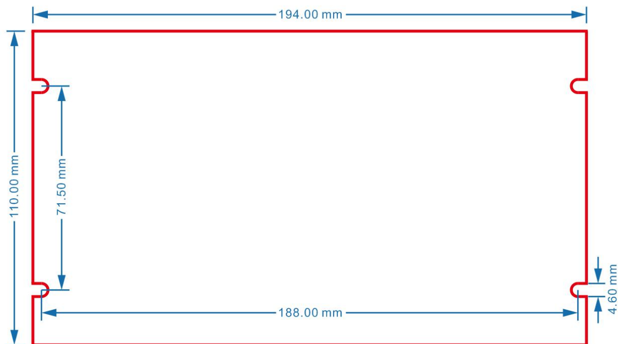
HK-3D-F00 尺寸图
