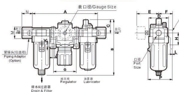
DAC3000~5000
