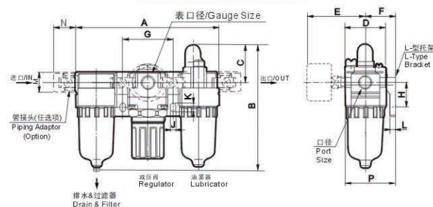
DAC1000~2000
