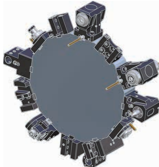
Doppel-Bohrstangenhalter double boring bar holder
