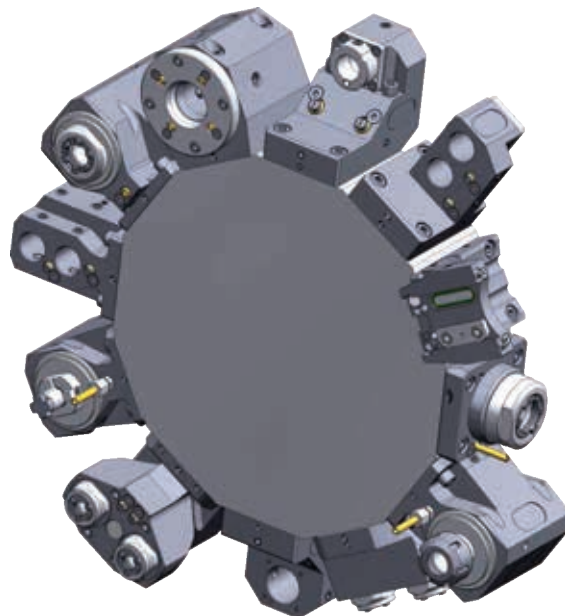
Doppel-Bohrstangenhalter double boring bar holder
