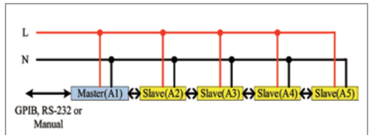
图10: 并联接法
