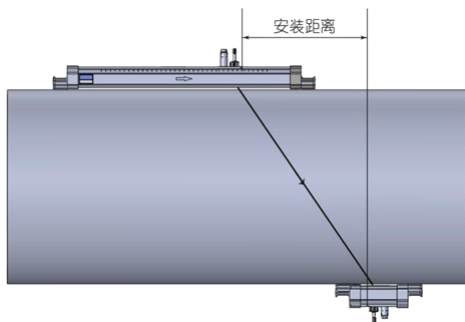
延长支架Z法安装俯视图
