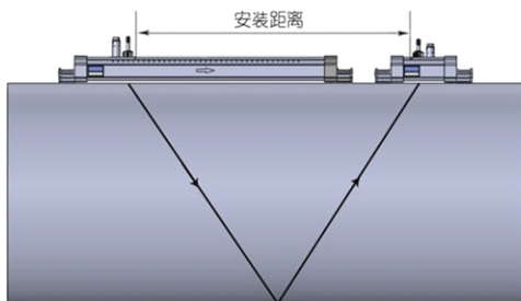
延长支架V法安装俯视图
