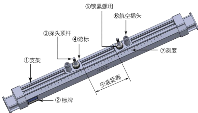
支架探头部件说明图 1
