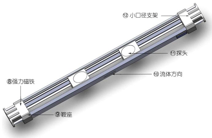
支架探头部件说明图 2
